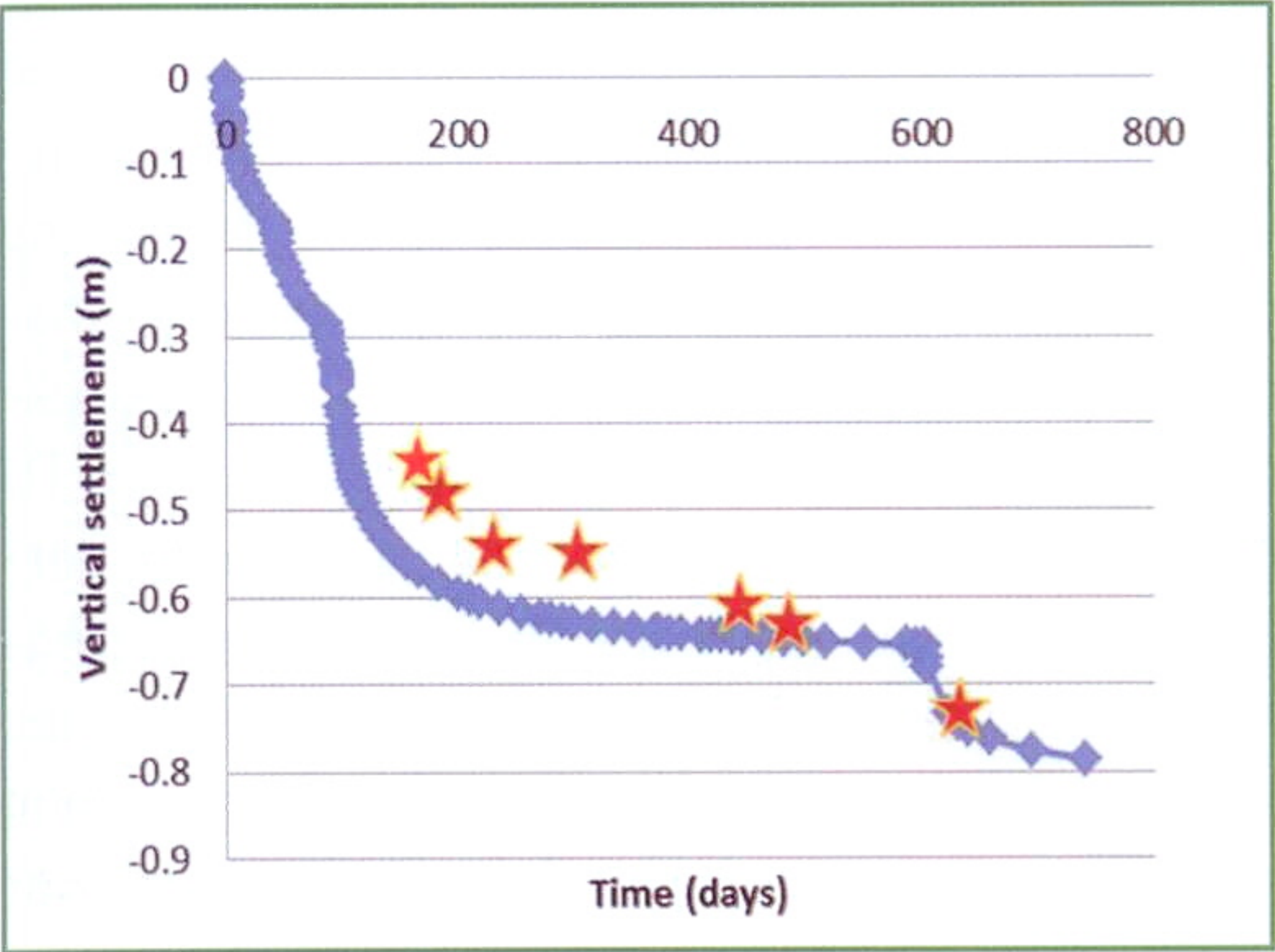
Figuur 2 - Middels zaakbakens gemeten zettingen versus het met Plaxis-model uitgerekende zettingverloop voor een dwarsprofiel van de N201
